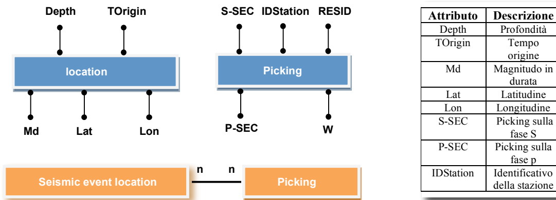
Figura 1. Sopra, entità impiegate nella modellizzazione del dato sismico. Sotto, relazione tra le entità. Nella tabella è riportata una descrizione esplicativa degli attributi mostrati in figura.
