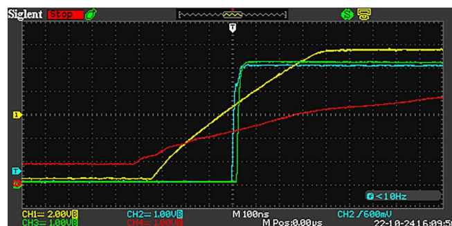
Figura 6 Segnali di sincronizzazione. La scala temporale con cui sono mostrati i segnali è stata impostata a 100 ns/div.
