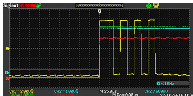
Figura 5 Segnali di sincronizzazione. La scala temporale con cui sono mostrati i segnali è stata impostata a 25 \mu\text{s}/\text{div} per mostrare l'intero byte seriale (CH1) trasmesso in corrispondenza del PPS.
