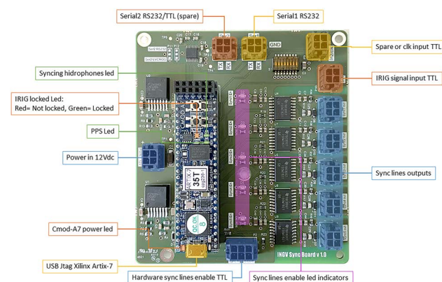
Figura 1 Syncboard e sue interfacce hardware.
