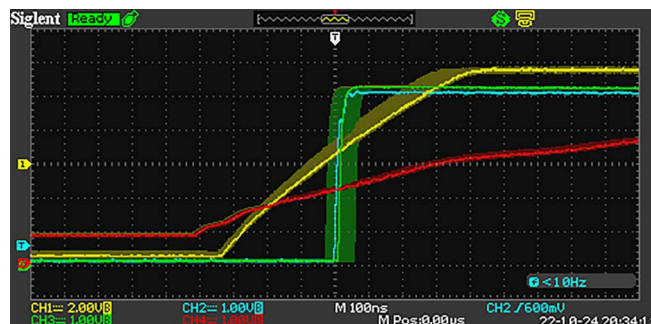
Figura 7 Jitter dei segnali di sincronizzazione della Syncboard rispetto al tempo GPS del laboratorio di terra. Figure 7 Jitter of Syncboard sync signals versus on-shore lab GPS time.
