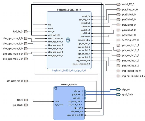
Figura 3 Architettura della logica programmabile. Figure 3 Programmable logic architecture.
