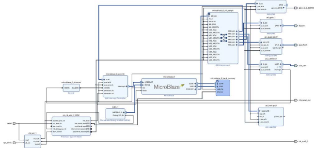
Figura 4 Dettaglio del modulo uBlaze_system . Figure 4 Detail of uBlaze_system module.
