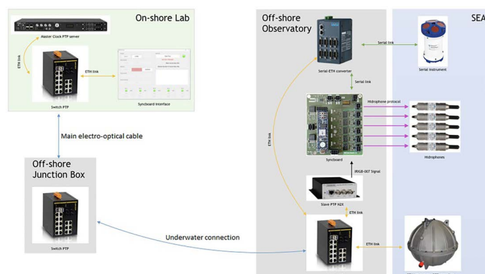
Figura 2 Schema di connessione dell'infrastruttura.
