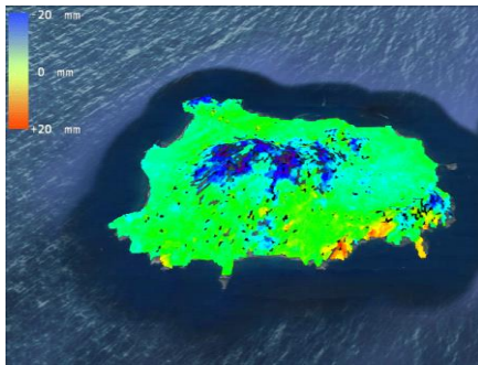
Figura 2.3.1 - a) mappa di deformazione, coppia 03.01.2020-25.06.2020, orbita ascendente, track 177, B.L=17.9m .
