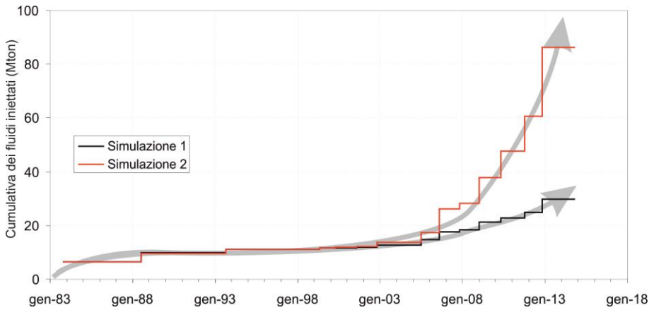
Figura 4.13 - Curve cumulative delle quantità di fluidi magmatici iniettati nel sistema idrotermale dei Campi Flegrei riferite alla simulazione 1 (Chiodini et al., 2012) e alla simulazione 2 (Chiodini et al., 2016). Per maggiori dettagli vedi il testo e i lavori citati.
