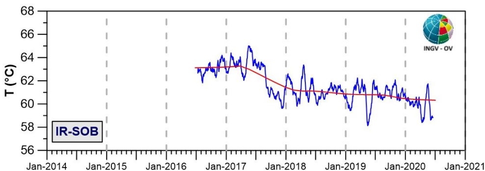
Figura 3.1.7 - Stazione IR-SOB. Serie temporali dei valori di temperatura massima rilevati nelle immagini IR: media mensile (blu), trend a lungo termine (rosso).
