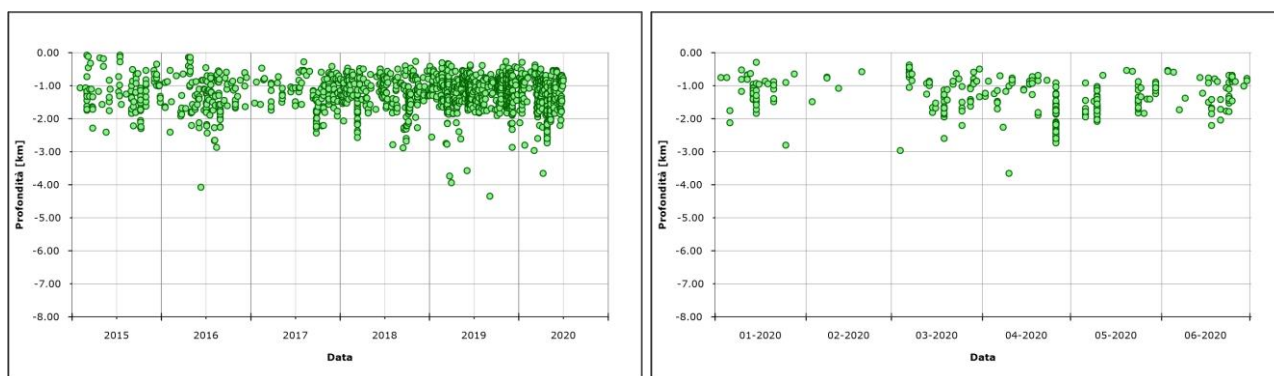
Figura 1.1.5 – Variazione temporale della profondità ipocentrale dei terremoti nell’area flegrea localizzati nel corso degli ultimi 5 anni (a sinistra) e del primo semestre 2020 (a destra).
