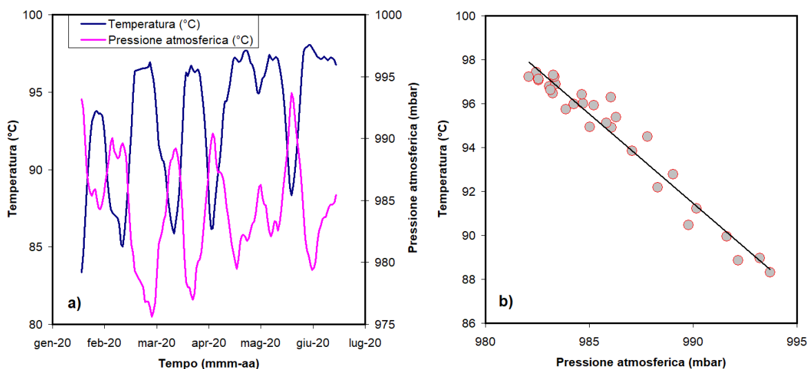
Figura 4.2.4 - a) Media mobile dei valori di temperatura dell'emissione fumarolica di Mt.Cito (Pizzone) e della pressione atmosferica misurati in continuo. La buona correlazione inversa dei due parametri è osservabile nel diagramma di destra (b).
