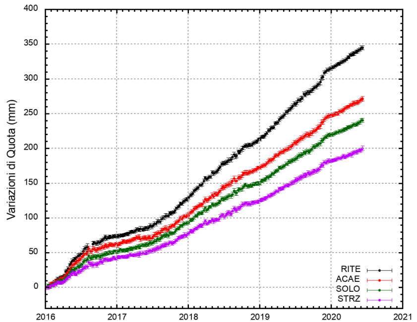
Figura 2.1.3 - Serie temporali delle variazioni in quota delle stazioni di RITE (Pozzuoli – Rione Terra), ACAE (Accademia Aeronautica), SOLO (Solfatar) e STRZ (Pozzuoli - Cimitero) da gennaio 2016 a giugno 2020.
