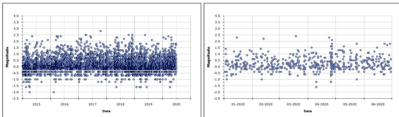
Figura 1.1.7 - Variazione temporale della magnitudo dei terremoti vesuviani nel corso degli ultimi 5 anni (a sinistra) e del primo semestre 2020 (a destra).
