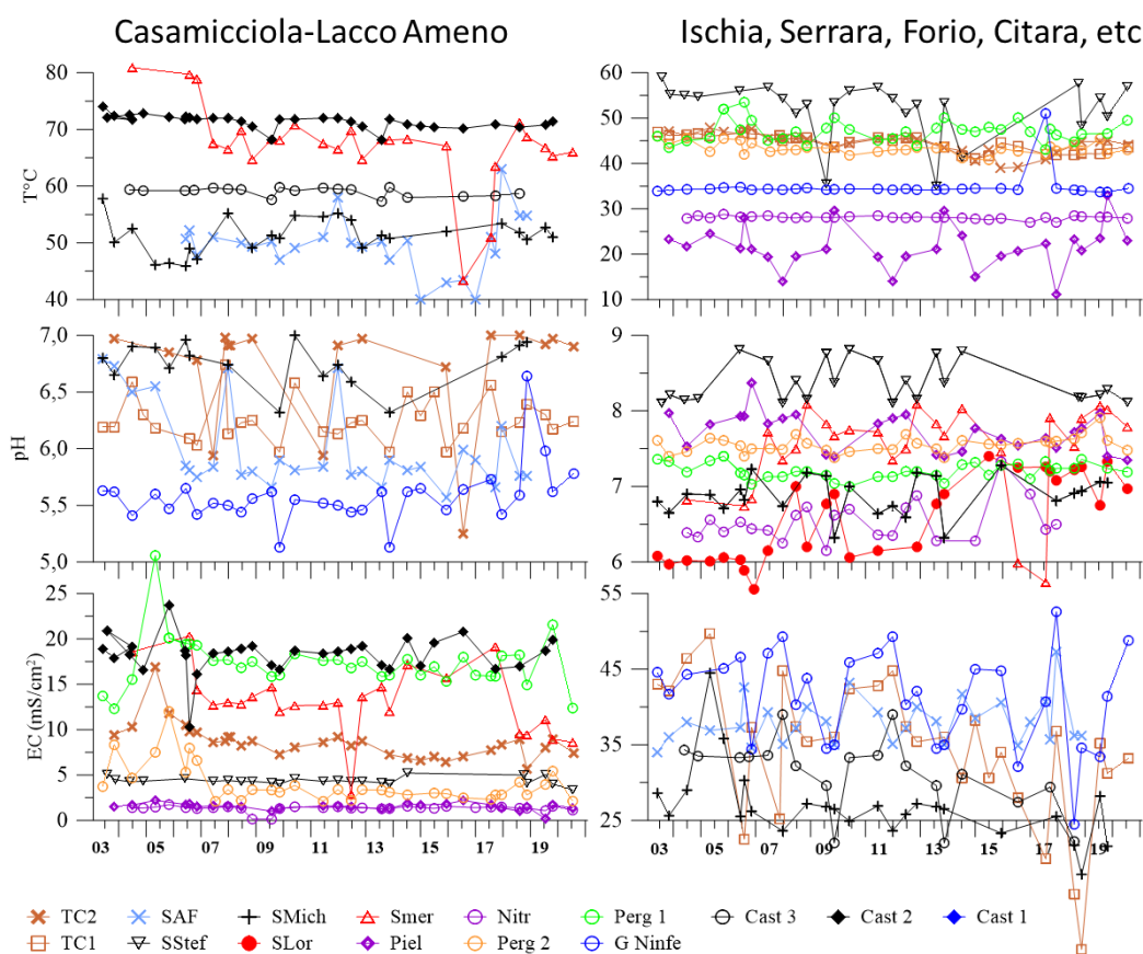
Figura 4.1.2 – Variazioni temporali di temperatura ( ^{\circ}C ), conducibilità ( mS/cm^2 ) e pH delle acque campionate.
