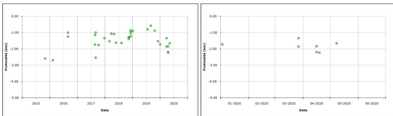
Figura 1.1.5 – Variazione temporale della profondità ipocentrale dei terremoti localizzati a Ischia nel corso degli ultimi 5 anni (a sinistra) e del primo semestre 2020 (a destra).
