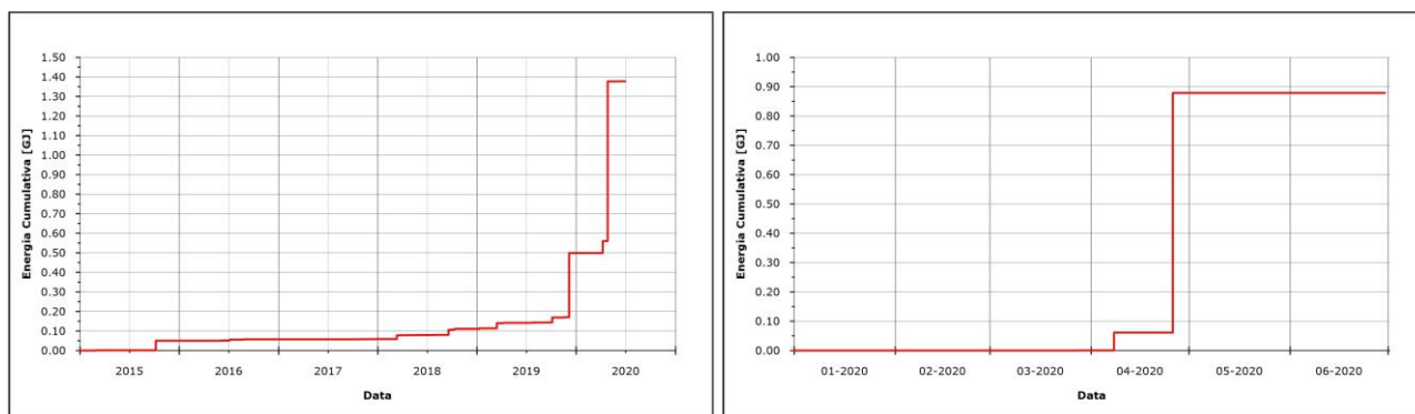
Figura 1.1.7 – Andamento cumulativo dell’energia rilasciata dai terremoti nell’area flegrea nel corso degli ultimi 5 anni (a sinistra) e del primo semestre 2020 (a destra) calcolato attraverso la relazione di Gutenberg-Richter \log E = 2.4 + 2.14 M - 0.054 M^2 .
