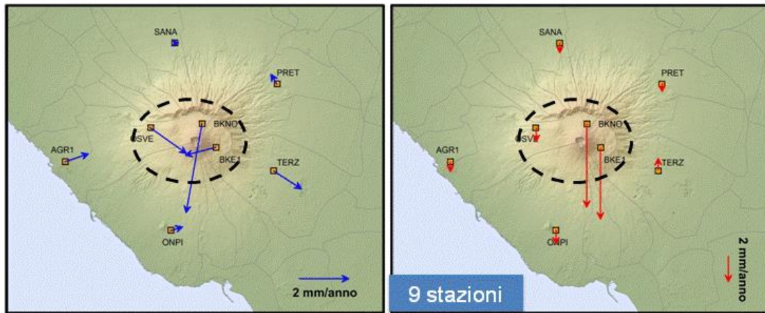
Figura 2.1.2 - Campo di velocità (in mm/anno) degli spostamenti orizzontali (in blu) e verticali (in rosso) nell'intervallo gennaio 2011-giugno 2020.
