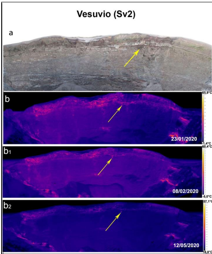
Figura 3.2.2 – Settore orientale del cratere del Vesuvio. Fotocomposizioni di immagini nel visibile (a) e delle corrispondenti immagini termiche relative al 23/01/2020 (b), 08/02/2020 (b1) e 12/05/2020 (b2) dal punto stazione SV2a di Fig. 3.2.1.
