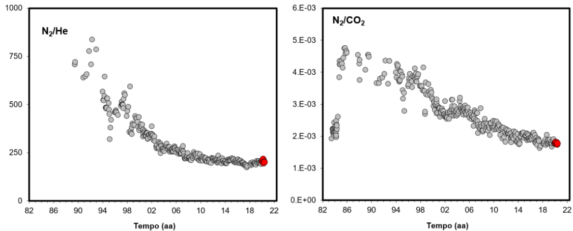
Figura 4.12 - Cronogramma dei rapporti N_2/He e N_2/CO_2 relativi alla fumarola BG. In rosso sono evidenziati i campioni del primo semestre 2020 che confermano i trend di diminuzione già identificati.
