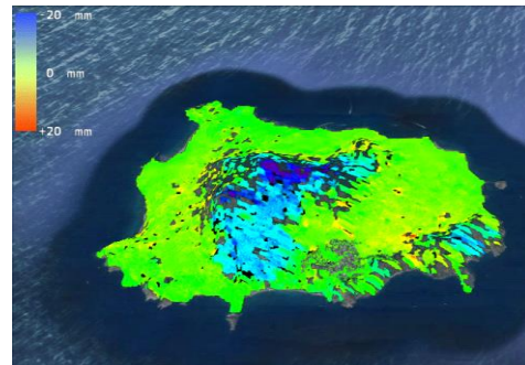
Figura 2.3.1 - b) mappa di deformazione, coppia 03.01.2020-25.06.2020, orbita discendente, track 22, B.L=19m .
