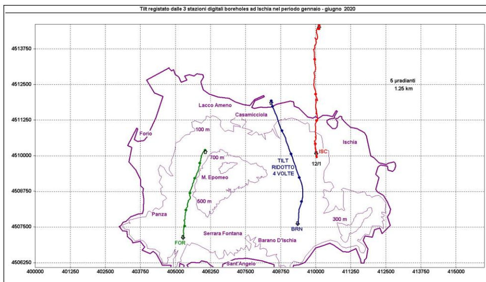
Figura 2.2.2 – Pattern tiltmetrico osservato ad Ischia. Il lato di ogni maglia del reticolo equivale a 5 \mu radianti o 1.25 km ed i pallini in colore sovrapposti sui vettori tilt indicano l'inizio di 30 giorni. Allo scopo di facilitare il confronto tra le varie stazioni, all'odografo relativo alla stazione BRN è stata applicata una scala di riduzione di 1:4.
