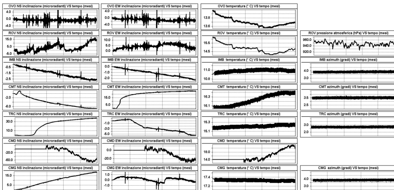
Figura 2.2.3 - Segnali registrati nei primi 6 mesi del 2020 dai 7 sensori analogici e digitali della rete del Vesuvio; le stazioni tiltmetriche sono ordinate dal basso verso l'alto secondo la latitudine. Le prime 2 colonne riportano le componenti NS ed EW in \mu radianti i cui valori di tilt crescenti nel tempo indicano rispettivamente la variazione di inclinazione del suolo a N e ad E. La terza colonna riporta le temperature in ^{\circ} C registrate da ogni sensore ed infine l'ultima colonna è riservata ai segnali non rilevati da tutte le stazioni, come la pressione atmosferica in hPa acquisita a ROV e la variazione di declinazione magnetica in gradi registrata dai sensori Lily. Per questi ultimi, la dicitura AzNW significa azimuth antiorario misurato dalla bussola a fondo pozzo.
