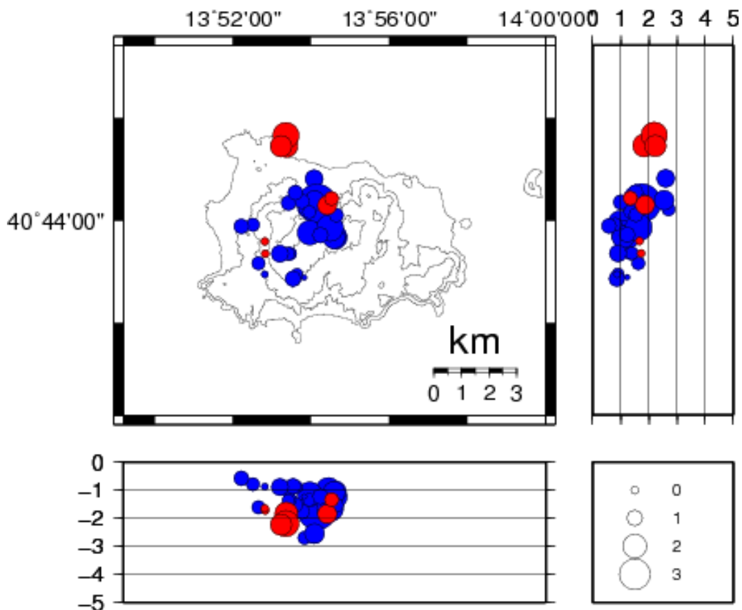
Figura 1.1.4 – Localizzazione degli ipocentri dei terremoti registrati ad Ischia nel corso degli ultimi 5 anni (in blu) e nel primo semestre 2020 (in rosso).
