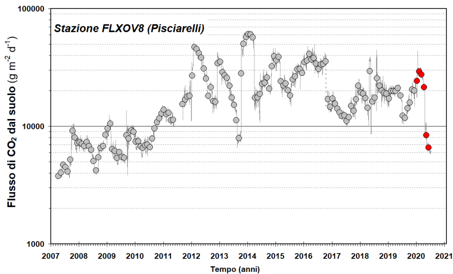
Figura 4.7 - Medie giornaliere (linea) e medie mensili (cerchi) dei flussi di CO 2 misurati a Pisciarelli (FLXOV8). I flussi di CO 2 dal suolo mostrano, in generale, un significativo incremento a partire dal 2010. In rosso sono evidenziate le medie mensili dei valori del primo semestre 2020. L'intervento di riparazione della stazione, effettuato nel mese di novembre 2016, per il ripristino del sistema per la misura del flusso di CO 2 dal suolo, ha comportato una modifica permanente del sito con valori misurati di flusso di CO 2 più bassi.
