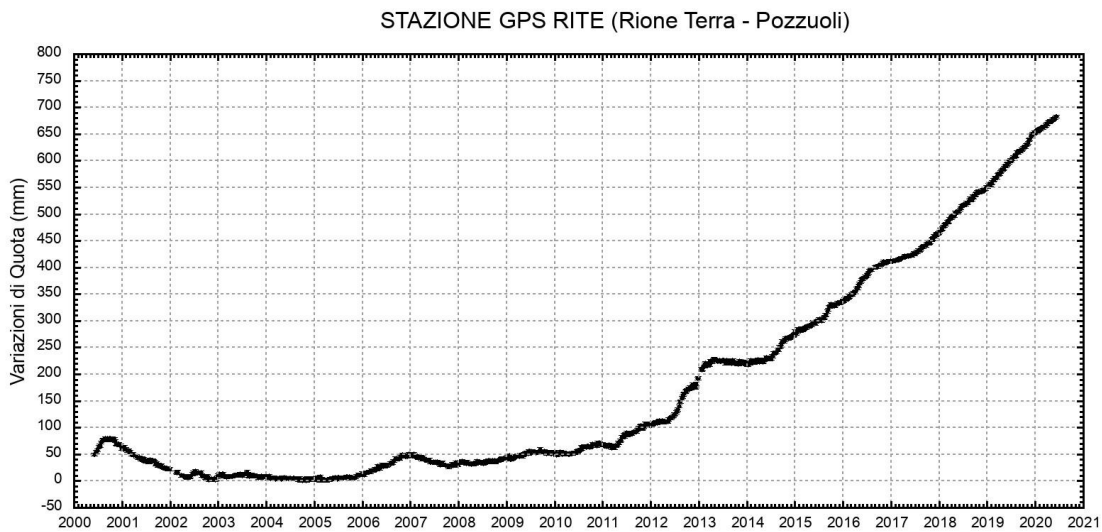
Figura 2.1.2 – Serie temporale delle variazioni in quota settimanali della stazione di RITE (Pozzuoli) dal 2000 a giugno 2020.
