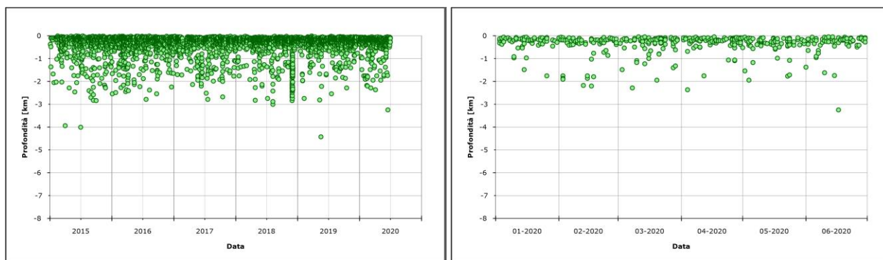
Figura 1.1.5 – Variazione temporale della profondità ipocentrale dei terremoti vesuviani localizzati nel corso degli ultimi 5 anni (a sinistra) e del primo semestre 2020 (a destra).
