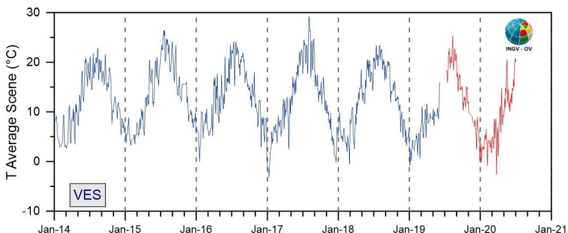
Figura 3.1.4 - Stazione Vesuvio: Serie temporale dei valori di temperatura media relativi ad ogni immagine acquisita con la precedente stazione (linea blu) e con quella di recente installazione (linea rossa).
