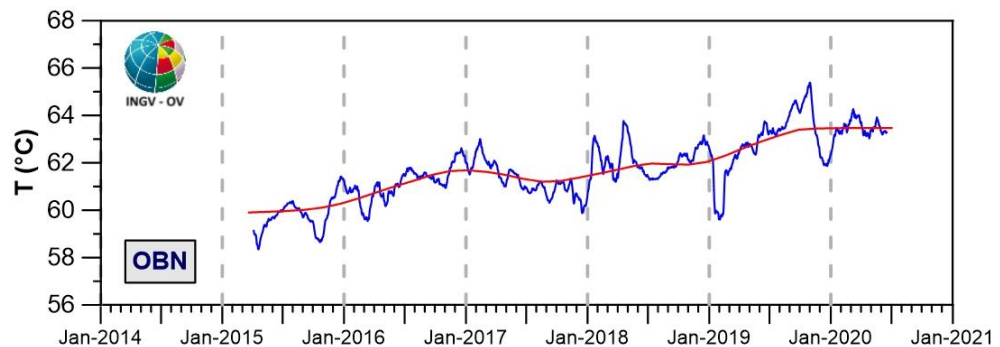
Figura 3.1.6 - Stazione Monte Olibano (OBN). Serie temporale delle medie mensili dei valori di temperatura massima rilevati nell'immagine IR destagionalizzata mediante applicazione dell'algoritmo STL.
