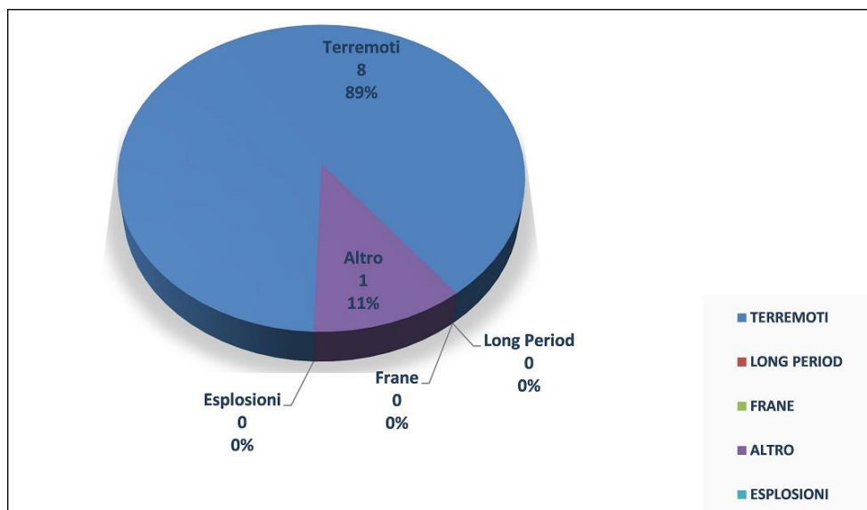
Figura 1.1.2 – Distribuzione percentuale degli eventi per tipologia nel primo semestre 2020.
