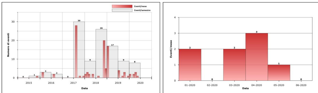
Figura 1.1.3 – Frequenza di accadimento dei terremoti registrati ad Ischia nel corso degli ultimi 5 anni (a sinistra) e del primo semestre 2020 (a destra).
