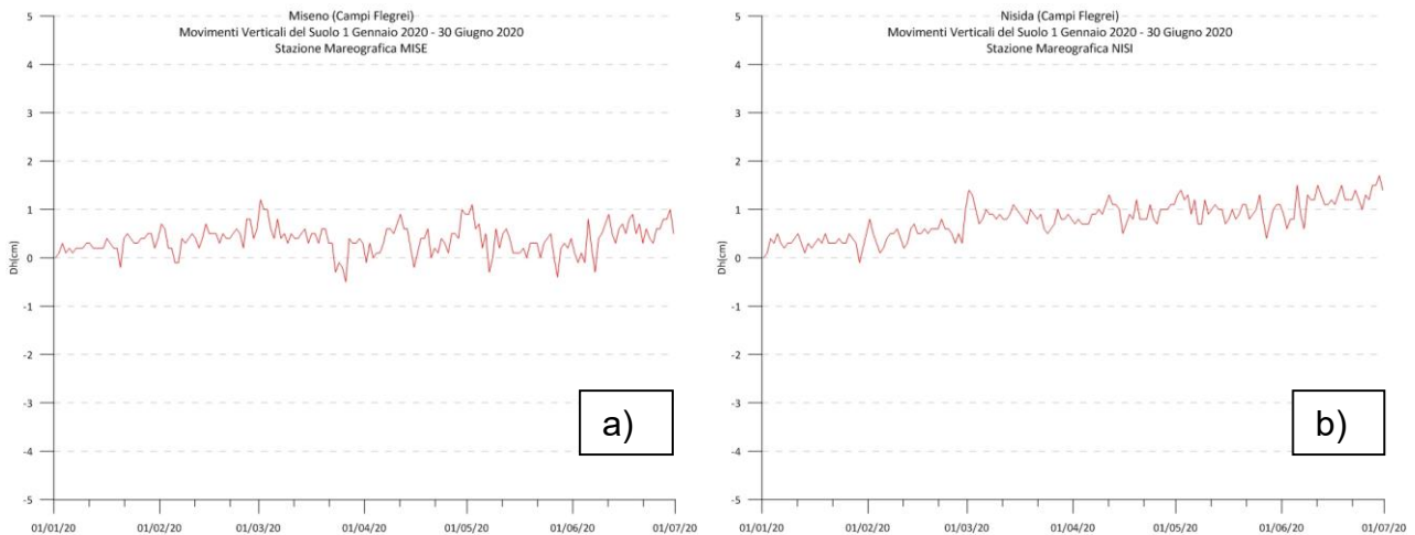
Figura 2.3.4 - Movimenti verticali del suolo, nel periodo gennaio 2020 – giugno 2020, ottenuti dall’analisi dei dati acquisiti da (a) sensore digitale alla stazione mareografica di Miseno (MISE) (bordo occidentale della caldera flegrea) e (b) alla stazione mareografica di Nisida (NISI) (bordo orientale della caldera flegrea). Le variazioni riportate rappresentano le medie giornaliere e sono riferite alla stazione di Napoli molo S.Vincenzo (NAMM).
