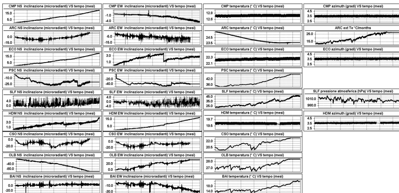
Figura 2.2.3 - Segnali registrati nei primi 6 mesi del 2020 da 9 dei 10 sensori della rete flegrea; le stazioni tiltmetriche sono ordinate dal basso verso l'alto secondo la latitudine. Le prime 2 colonne riportano le componenti NS ed EW in \mu radianti i cui valori di tilt crescenti nel tempo indicano la variazione di inclinazione del suolo a N e ad E. La terza colonna riporta le temperature in °C registrate da ogni sensore ed infine l'ultima colonna è riservata ai segnali non rilevati da tutte le stazioni, come la temperatura misurata a bocca pozzo ad ARC, la pressione atmosferica in hPa acquisita a SLF e la variazione di declinazione magnetica in gradi registrata dai sensori Lily. Per questi ultimi, la dicitura AzNW significa azimuth antiorario misurato dalla bussola a fondo pozzo.
