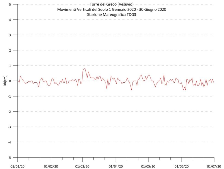
Figura 2.3.2 - Movimenti verticali del suolo, nel periodo gennaio 2020 – giugno 2020, ottenuti dall'analisi dei dati acquisiti dal sensore digitale alla stazione mareografica di Torre del Greco (TDG3). Le variazioni riportate rappresentano le medie giornaliere e sono riferite alla stazione di Napoli Molo S.Vincenzo (NAMM).
