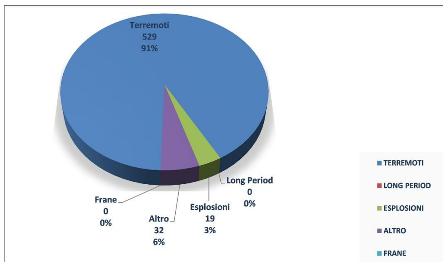
Figura 1.1.2 – Distribuzione percentuale degli eventi per tipologia nel primo semestre 2020. Le esplosioni riportate sono tutte di origine artificiale.
