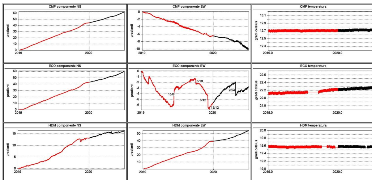
Figura 2.2.4 - Serie temporali dei segnali registrati a partire dal 2019 dalle 3 stazioni "borehole" della rete flegrea ordinate dal basso verso l'alto secondo la latitudine. Le prime 2 colonne riportano le componenti NS ed EW in \mu radianti i cui valori di tilt crescenti nel tempo indicano rispettivamente la variazione di inclinazione del suolo a N e ad E, mentre la terza colonna riporta la temperatura in ^{\circ} C registrata da ogni sensore. In rosso sono riportati i segnali relativi al 2019 mentre in nero sono rappresentati quelli registrati nel 2020. Le date annotate sul segnale EW di ECO indicano le maggiori variazioni tiltmetriche registrate, 3 delle quali sono state prodotte dai terremoti di maggiore energia occorsi nel 2019 (5/10 e 6/12) ed in questo anno (26/4).
