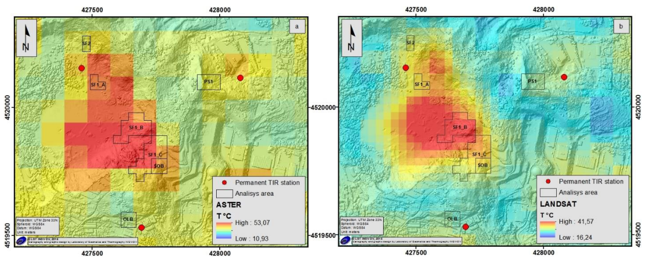
Figura 3.3.3 - Immagini termiche satellitari ASTER (a) e Landsat8 (b) rispettivamente del 22 e del 30 giugno 2020. I poligoni racchiudono le aree inquadrare dalla TIRNet.
