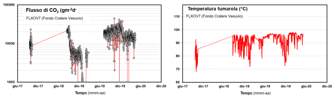
Figura 4.1.6 - Parametri misurati dalla stazione geochimica (FLXOV7) installata in area di fondo cratere del Vesuvio. I valori, eccetto il flusso di CO 2 dal suolo, sono riportati come medie giornaliere.
