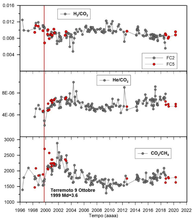
Figura 4.1.2 - Variazioni composizionali delle fumarole FC2 (simboli grigi) e FC5 (simboli rossi) nel periodo 1996-2020.
