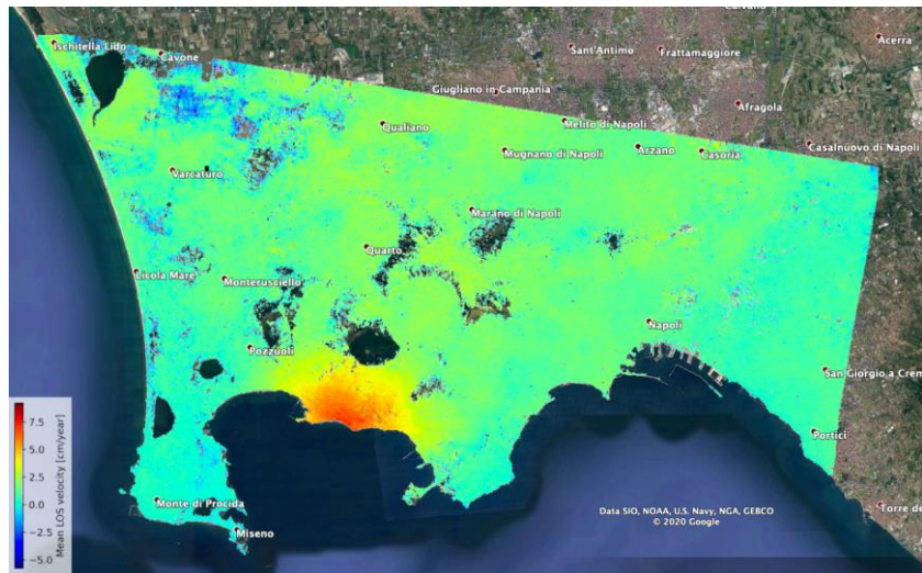
Figura 2.4.1 - Mappa della velocità media di deformazione nella linea di vista del sensore (Sentinel-1A/B) (03.01.2020-25.06.2020) per l'area Flegrea. Dati IWS - TOPS mode, orbite discendenti (22), swath 1.
