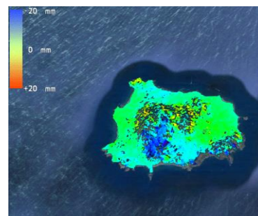
Figura 2.3.2 - b) componente orizzontale stimata a partire dai risultati mostrati in Fig.3.2.1a,b.
