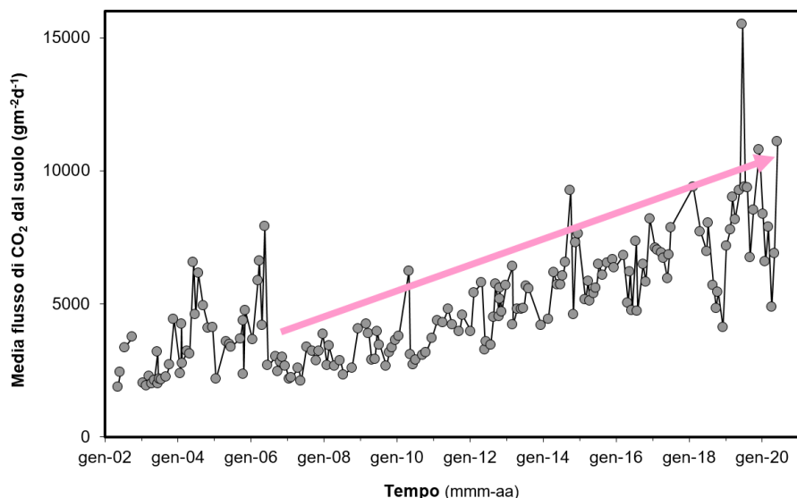
Figura 4.2 - Cronogramma della media dei flussi di CO 2 dal suolo misurati su ~60 punti fissi nell'area craterica della Solfatara.
