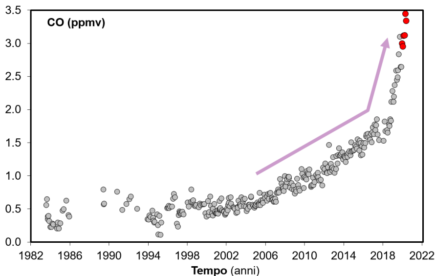
Figura 4.9 - Variazioni della concentrazione di monossido di carbonio (CO) misurato alla fumarola BG a partire dal 1983. In rosso sono evidenziati i campioni relativi al primo semestre 2020. In generale alti contenuti di CO caratterizzano sistemi vulcanici ad elevata temperatura mentre fumarole alimentate da sistemi idrotermali mostrano concentrazioni più basse, in tali sistemi un aumento delle concentrazioni di CO può riflettere un incremento delle condizioni di temperatura e pressione.
