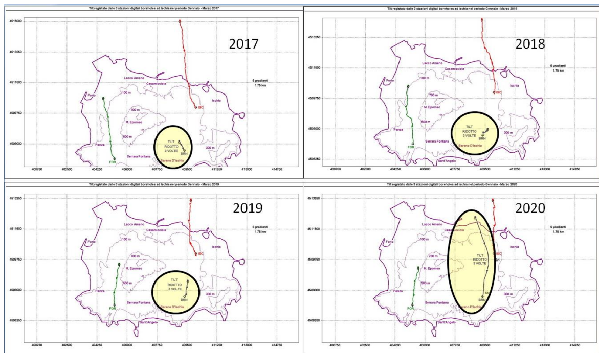
Figura 2.2.4 - Pattern tiltmetrico osservato ad Ischia nei primi 3 mesi del 2017, 2018, 2019 e 2020. Per agevolare il confronto è stata applicata una scala di riduzione di 1:3 all’odografo relativo alla stazione BRN. È evidente come nel corso di quest’anno l’ampiezza dell’inclinazione del suolo sia triplicata in corrispondenza del sito-stazione.
