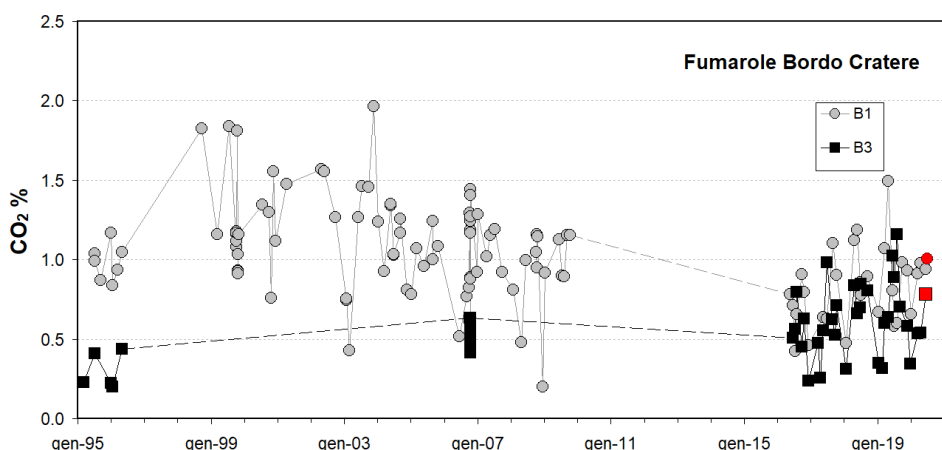
Figura 4.1.4 - Variazione temporale della concentrazione di CO_2 delle fumarole di bordo cratere). Con i simboli rossi sono riportati i campioni relativi al primo semestre 2020.
