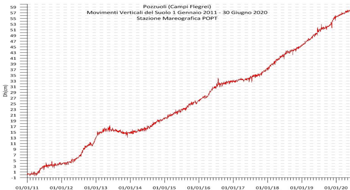
Figura 2.3.2 - Movimenti verticali del suolo, nel periodo gennaio 2011 - giugno 2020, ottenuti dall'analisi dei dati acquisiti dal sensore digitale alla stazione mareografica di Pozzuoli Porto (POPT) (area centrale della caldera flegrea). Le variazioni riportate rappresentano le medie giornaliere e sono riferite alla stazione di Napoli Molo S.Vincenzo (NAMM).
