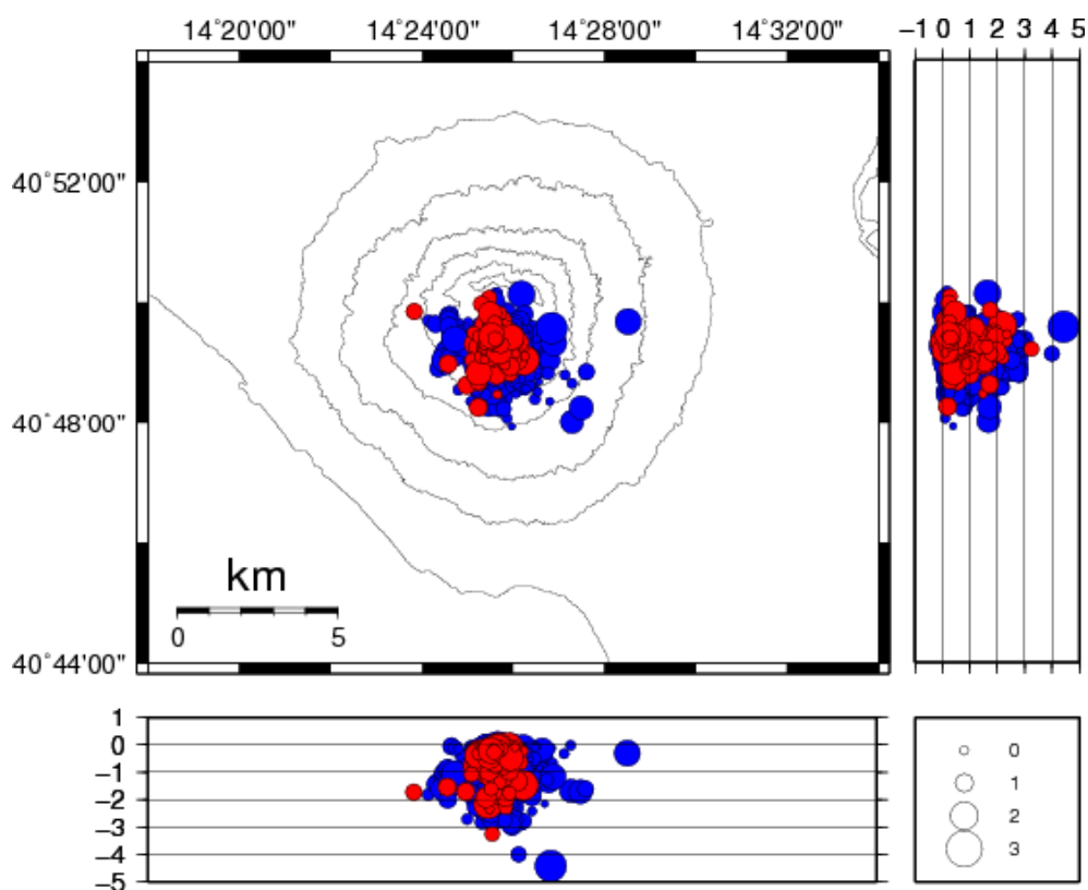
Figura 1.1.4 – Localizzazione degli ipocentri nell'area vesuviana durante gli ultimi 5 anni (in blu) e nel primo semestre 2020 (in rosso).
