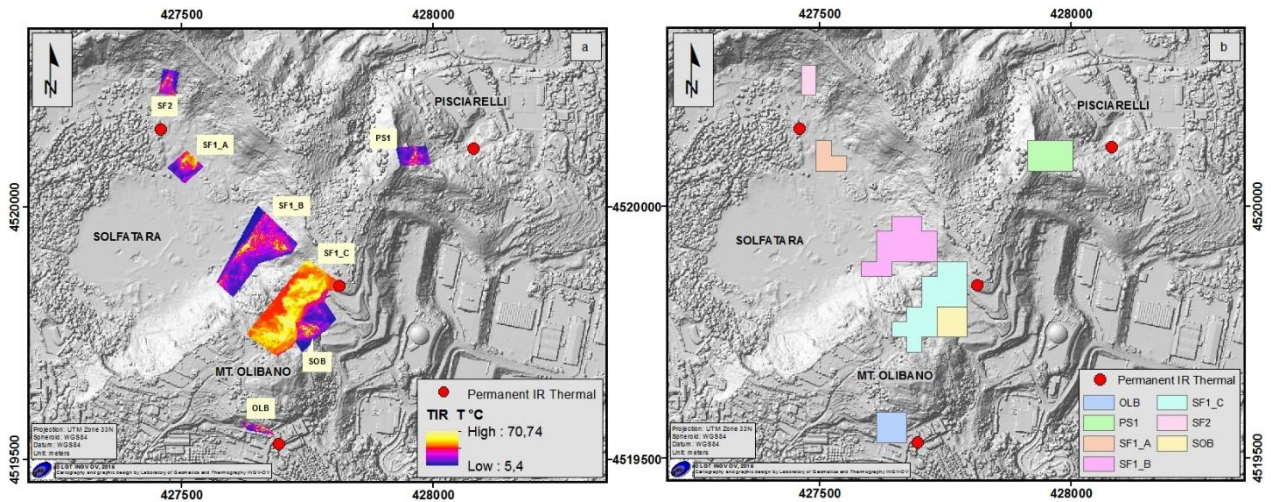
Figura 3.3.2 - Immagini termiche georiferite del 30/06/2020 (a) e aree di analisi (b).
