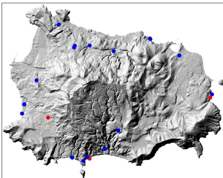
Figura 4.1.1 – Ubicazione dei punti di campionamento: blu = acque, rosso = gas liberi.
