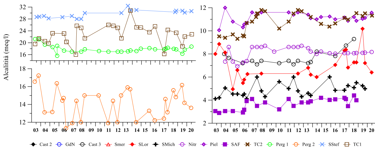
Figura 4.1.3 - Variazione temporale di alcalinità nelle acque campionate.
