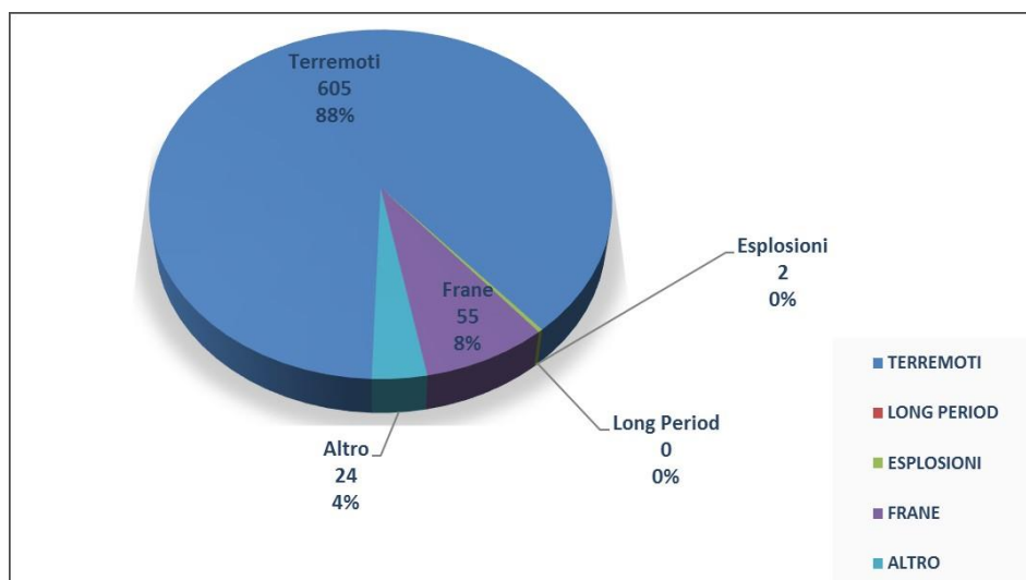
Figura 1.1.2 – Distribuzione percentuale degli eventi per tipologia nel primo semestre 2020. Le esplosioni riportate sono tutte di origine artificiale.
