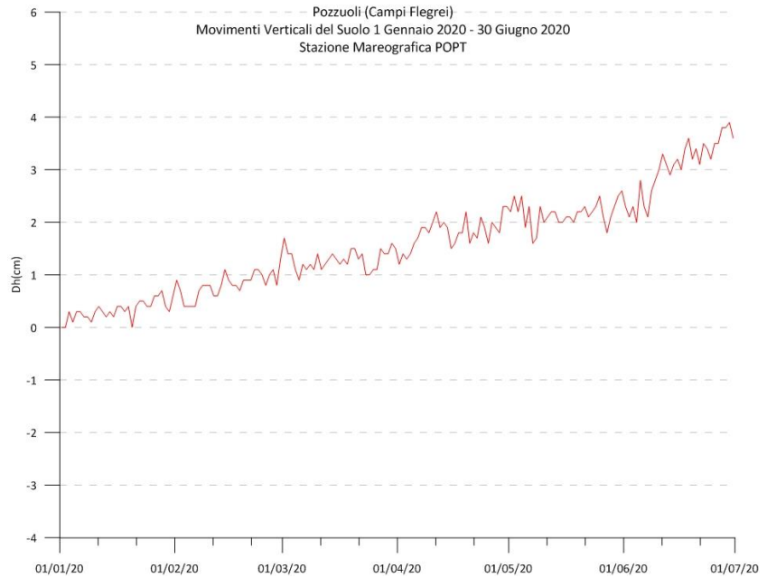
Figura 2.3.3 - Movimenti verticali del suolo, nel periodo gennaio 2020 – giugno 2020, ottenuti dall’analisi dei dati acquisiti dal sensore digitale alla stazione mareografica di Pozzuoli Porto (POPT) (area centrale della caldera flegrea). Le variazioni riportate rappresentano le medie giornaliere e sono riferite alla stazione di Napoli molo S.Vincenzo (NAMM).
