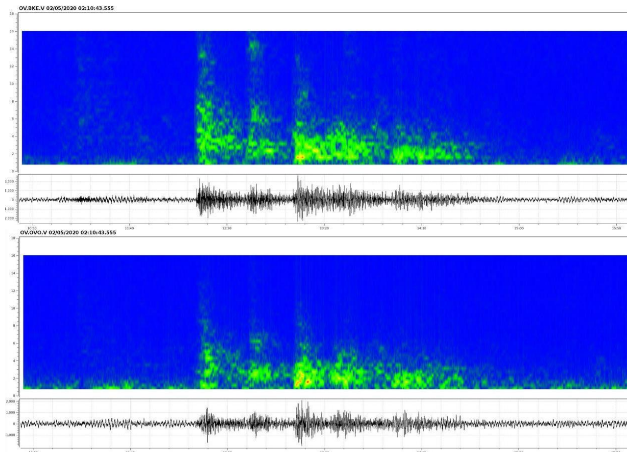
Figura 1.1.6 – Spettrogrammi degli eventi registrati il 02/05 alle stazioni di Bunker Est (BKE), in alto, e Osservatorio Vesuviano (OVO), in basso.
