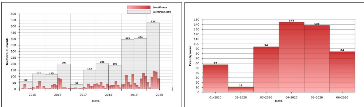
Figura 1.1.3 – Frequenza di accadimento dei terremoti ai Campi Flegrei nel corso degli ultimi 5 anni (a sinistra) e del primo semestre 2020 (a destra).
