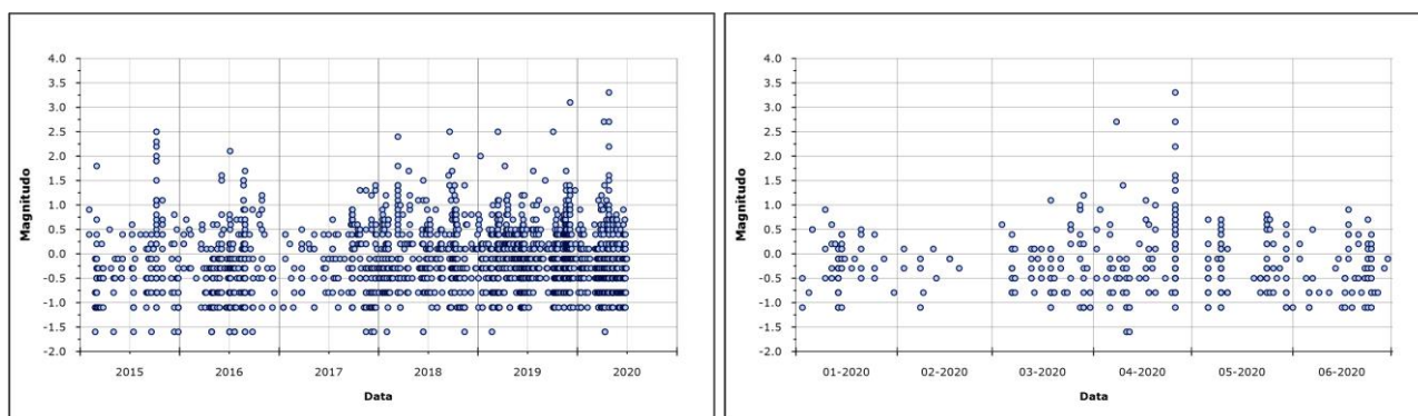
Figura 1.1.6 - Variazione temporale della magnitudo dei terremoti nell’area flegrea nel corso degli ultimi 5 anni (a sinistra) e del primo semestre 2020 (a destra).
