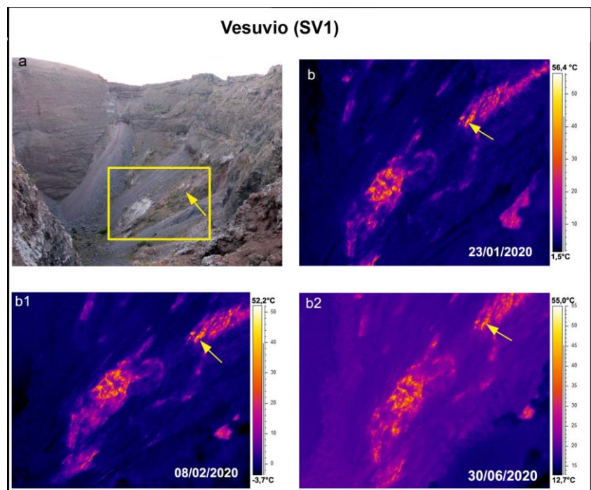
Figura 3.2.3 – Settore meridionale del cratere del Vesuvio. Immagini nel visibile (a) e immagini termiche, relative all'area ricadente nel riquadro giallo (a), riprese il 23/01/2020 (b), il 08/02/2020 (b1) e il 30/06/2020 (b2) dal punto stazione SV1 di Figura 3.2.1; la freccia gialla indica l'area che costantemente è a più alta temperatura.
