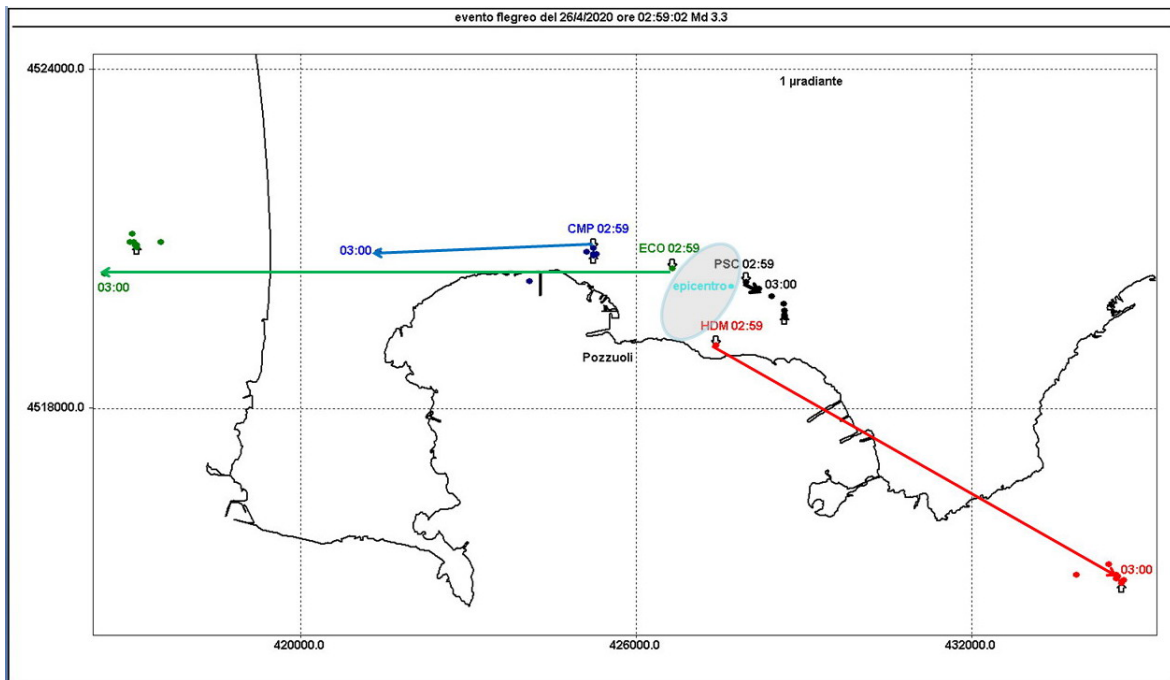
Figura 2.2.5 - Pattern tiltmetrico osservato ai Campi Flegrei nei primi 9 minuti, compreso quello dell'evento. È riportato con un pallino colorato sia l'epicentro che la proiezione in superficie del centroide di deformazione ipotizzato.
