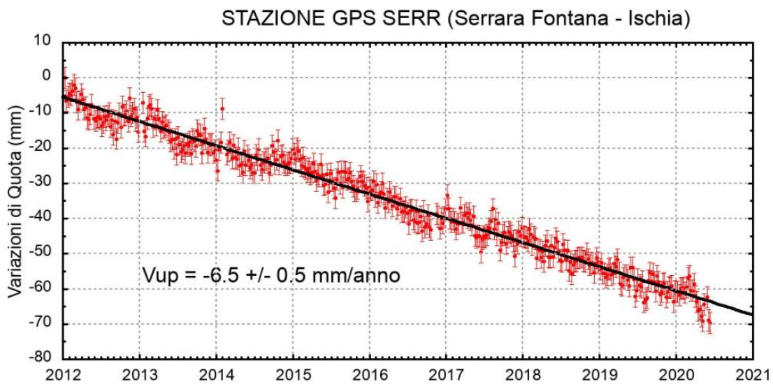
Figura 2.1.3 - Serie temporale delle variazioni settimanali in quota della stazione di SERR (Ischia) da gennaio 2012 a giugno 2020.
