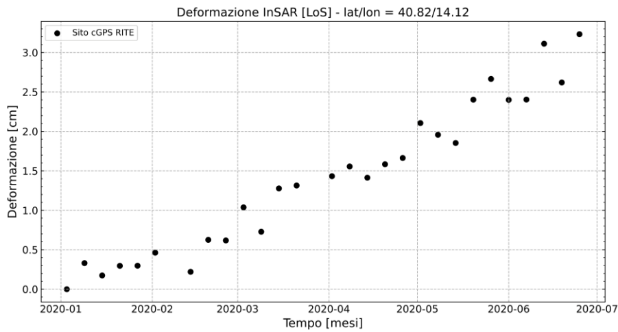
Figura 2.4.2 - Serie temporale (03.01.2020-25.06.2020) estratta in corrispondenza della stazione GPS in continuo RITE nell'area di massima deformazione.
