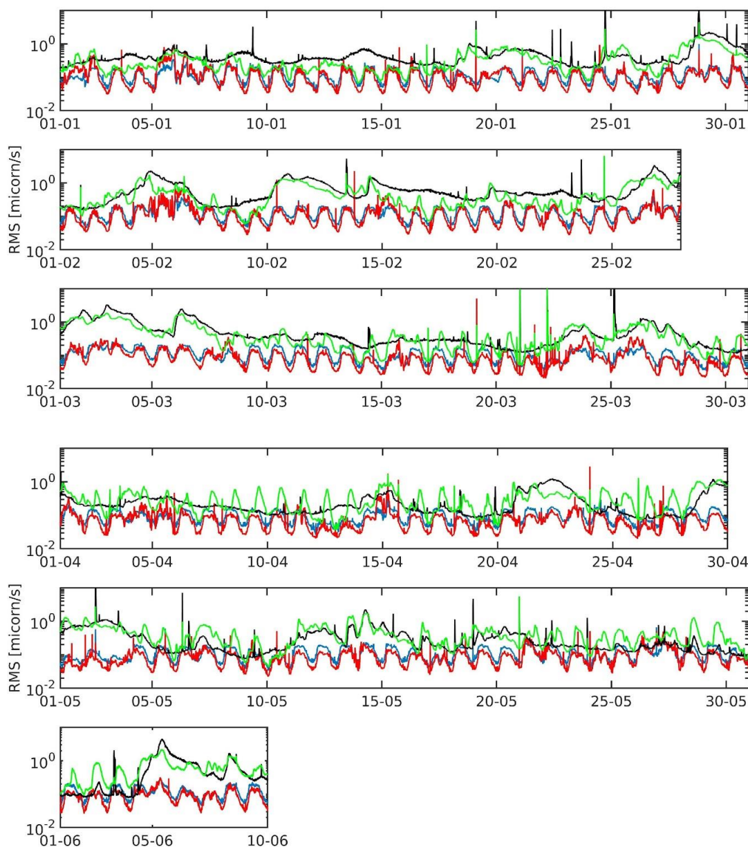
Figura 1.2.2 - RMS calcolato per i segnali della stazione sismica BKWG nel primo semestre del 2020 in quattro bande di frequenza: 0.05-0.5 Hz (nero), 0.5-2 Hz (verde), 2-4 Hz (rosso), 4-8 Hz (blu).
