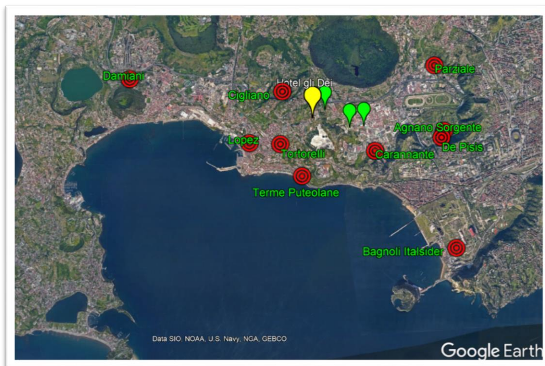
Figura 4.17 - Ubicazione dei punti di misura e campionamento delle acque di falda relativi alla campagna del 2020, con il simbolo rosso sono riportati i siti della rete di monitoraggio multiparametrico in continuo della falda. In giallo la prima stazione equipaggiata con i nuovi sensori HT (fino a 100 °C).
