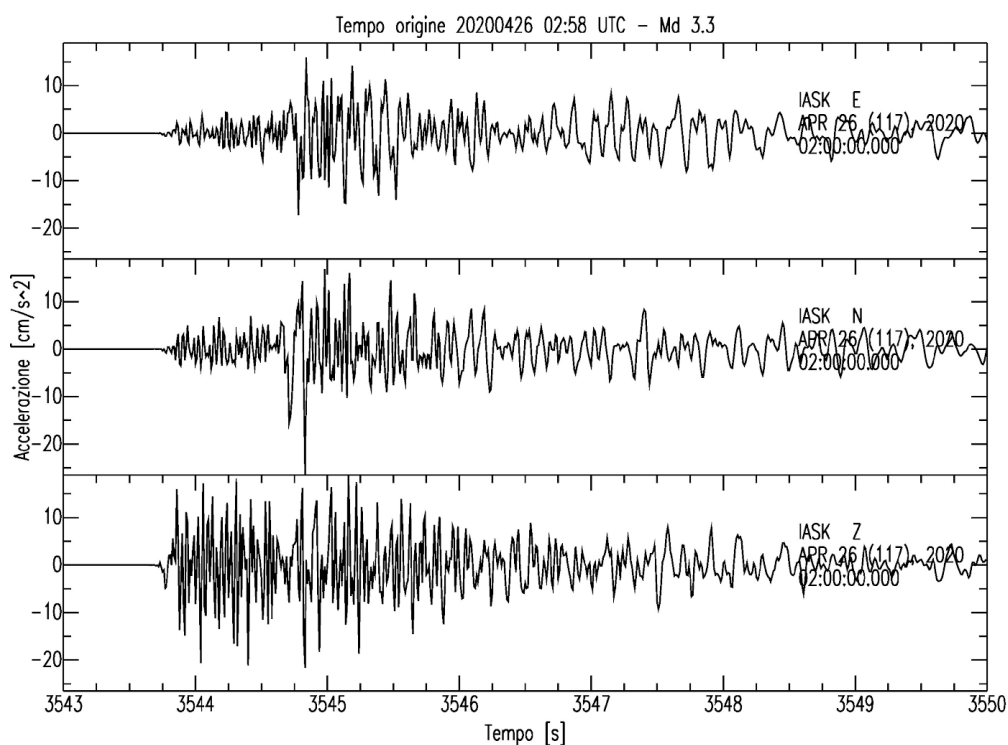
Figura 1.2.5 - Accelerogramma della stazione IASK per il terremoto M_d=3.3 202004260258 avvenuto nell'area dei Campi Flegrei.
