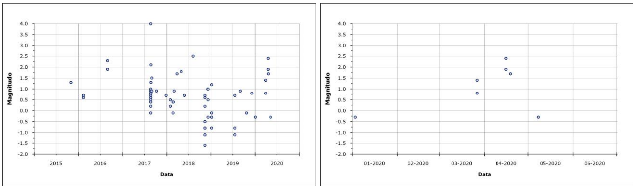
Figura 1.1.6 - Variazione temporale della magnitudo dei terremoti registrati ad Ischia nel corso degli ultimi 5 anni (a sinistra) e del primo semestre 2020 (a destra).
