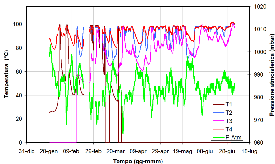
Figura 4.2.3 - Temperature misurate in continuo dell'emissione fumarolica di Mt.Cito (Pizzone), e di altri punti limitrofi, la pressione atmosferica è stata inclusa tra i parametri monitorati.
