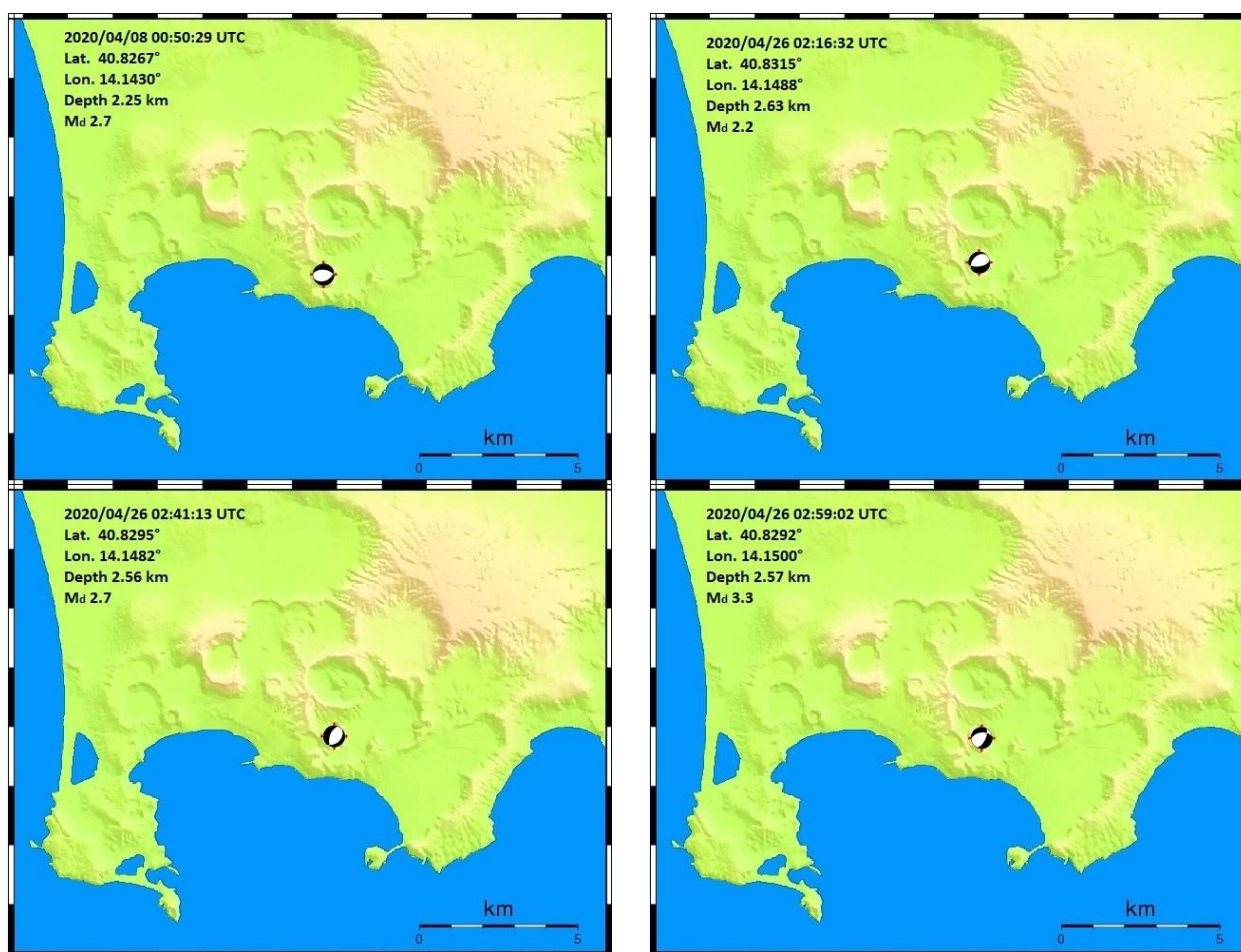
Figura 1.1.8 - Meccanismi focali elaborati per eventi di magnitudo > 1.5 registrati ai Campi Flegrei nel primo semestre 2020.
