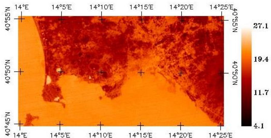
Figura 3.3.4 - Mappa di temperatura superficiale relativa al dato ASTER acquisito alle 21.10 UTC del 28 maggio 2020.
