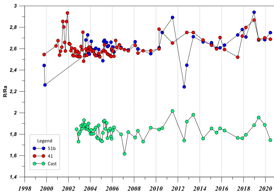
Figura 4.2.6 – Variazione temporale del rapporto R/Ra nelle acque sotterranee.
