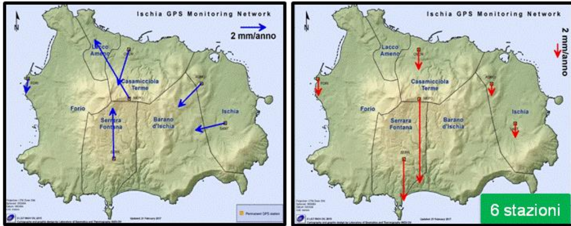
Figura 2.1.2 - Campo di velocità (in mm/anno) degli spostamenti orizzontali (in blu) e verticali (in rosso) nell'intervallo gennaio 2011 - giugno 2020.
