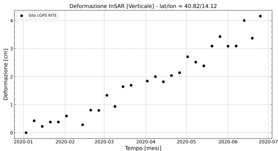
Figura 2.4.4 - Serie temporale (03.01.2020-25.06.2020) estratta in corrispondenza della stazione GPS in continuo RITE; dato in linea di vista ridotto alla verticale.
