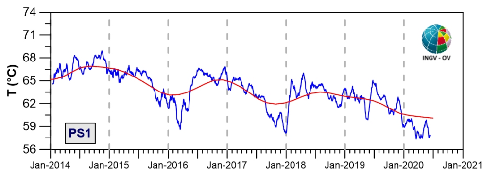
Figura 3.1.2 - Stazione Pisciarelli (PS1). Serie temporali dei valori di temperatura massima rilevati nelle immagini IR: media mensile (blu), trend a lungo termine (rosso).
