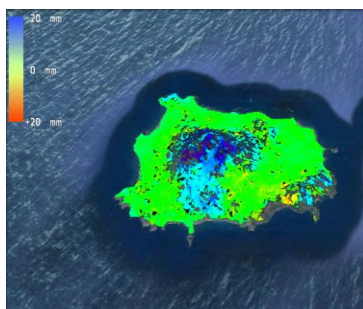
Figura 2.3.2 - a) componente verticale stimata a partire dai risultati mostrati in Fig.3.2.1a,b.
