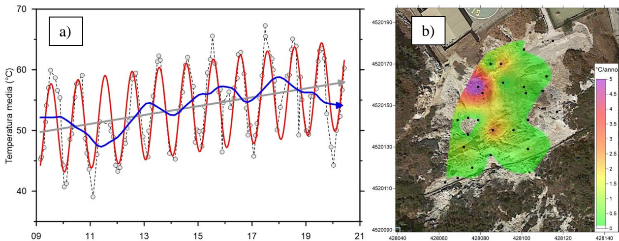
Figura 4.5 - Cronogramma della media delle temperature del suolo (a 10 cm di profondità) misurate su 25 punti fissi nell'area di Pisciarelli dal 2009. Il trend destagionalizzato, mediante l'utilizzo dell'algoritmo di destagionalizzazione STL (Seasonal-Trend decomposition based on Loess, Cleveland et al., 1990), è riportato con la linea blu.
