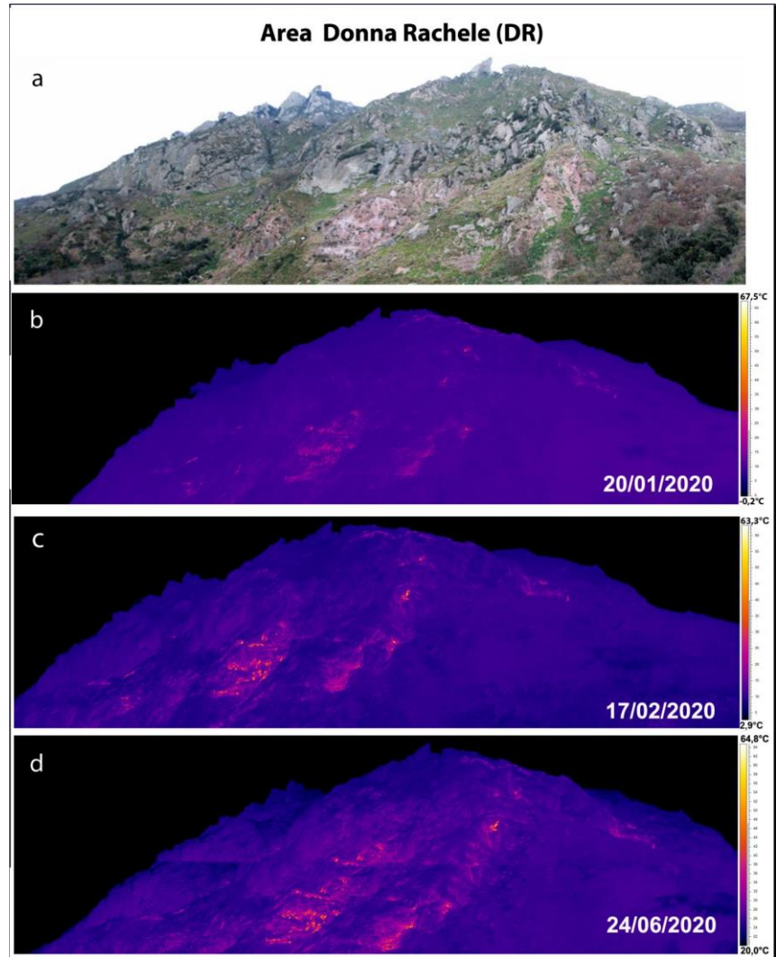
Figura 3.2 - Versante in località Donna Rachele a Ischia. Fotocomposizioni di immagini nel visibile (a) e delle corrispondenti immagini termiche relative al 20/01/2020 (b), 17/02/2020 (c) e 24/06/2020 (d) dal punto stazione DRp di figura 3.1.
