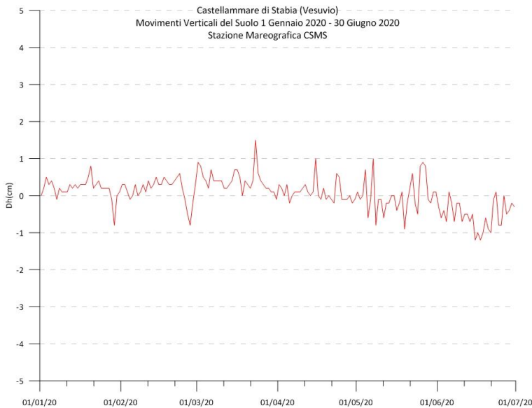
Figura 2.3.3 - Movimenti verticali del suolo, nel periodo gennaio 2020 – giugno 2020, ottenuti dall'analisi dei dati acquisiti dal sensore digitale alla stazione mareografica di Castellammare di Stabia (CSMS). Le variazioni riportate rappresentano le medie giornaliere e sono riferite alla stazione Napoli Molo S.Vincenzo (NAMM).
