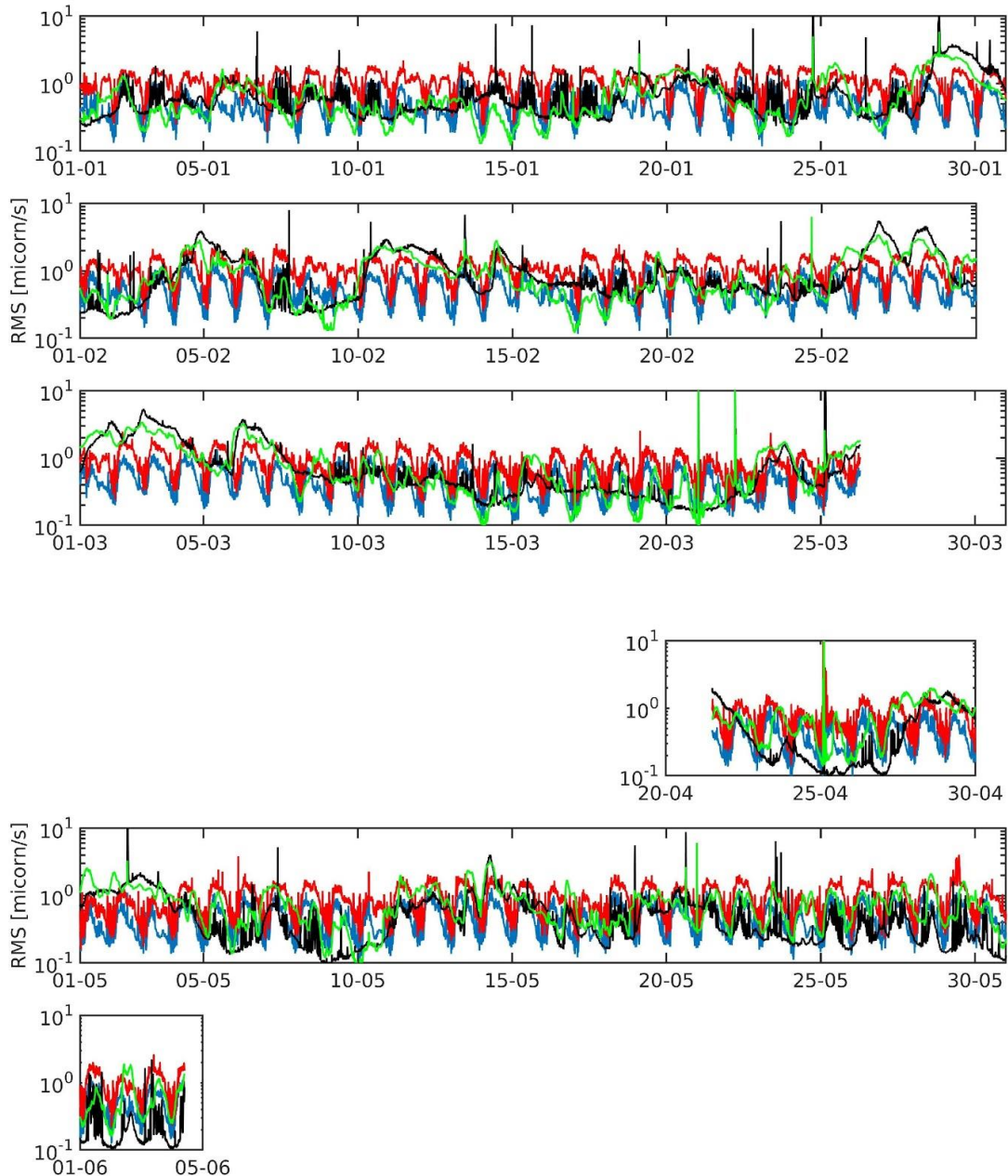
Figura 1.2.2 - RMS calcolato per i segnali della stazione sismica PESH nei primi sei mesi del 2020 in quattro bande di frequenza: 0.05-0.5 Hz (nero), 0.5-2 Hz (verde), 2-4 Hz (rosso), 4-8 Hz (blu). La mancanza presente tra il giorno 01 aprile e 22 aprile è stata causata da un problema al sistema di alimentazione.
