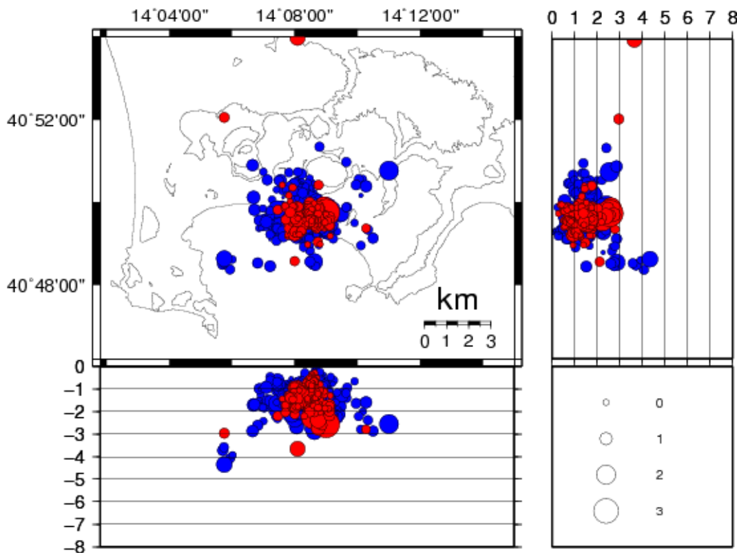
Figura 1.1.4 – Localizzazione degli ipocentri nell’area flegrea durante gli ultimi 5 anni (in blu) e nel primo semestre 2020 (in rosso).
