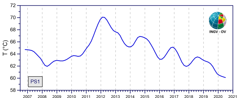
Figura 3.1.3 - Stazione Pisciarelli (PS1). Trend a lungo termine dei valori di temperatura massima rilevati nell'immagine IR ottenuto mediante applicazione dell'algoritmo STL.
