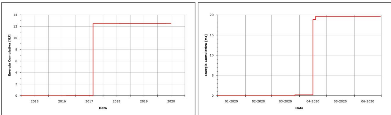
Figura 1.1.7 – Andamento cumulativo dell’energia rilasciata dai terremoti registrati ad Ischia nel corso degli ultimi 5 anni (a sinistra) e del primo semestre 2020 (a destra) calcolato attraverso la relazione di Gutenberg-Richter \log E = 2.4 + 2.14M - 0.054M^2 .
