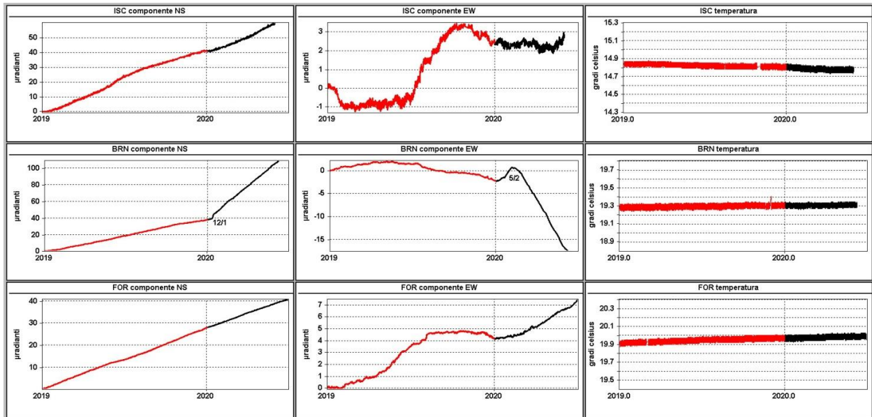
Figura 2.2.3 - Serie temporali dei segnali registrati a partire dal 2019 dalle 3 stazioni “borehole” della rete di Ischia ordinate dal basso verso l’alto secondo la latitudine. Le prime 2 colonne riportano le componenti NS ed EW in \mu radianti i cui valori di tilt crescenti nel tempo indicano rispettivamente la variazione di inclinazione del suolo a N e ad E, mentre la terza colonna riporta la temperatura in ^{\circ} C registrata da ogni sensore. In rosso sono riportati i segnali relativi al 2019 mentre in nero sono rappresentati quelli registrati nel 2020. Le date annotate sui segnali di BRN indicano l’improvvisa variazione di trend che ha interessato la stazione all’inizio del 2020.
