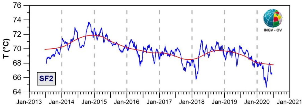
Figura 3.1.5 - Stazione Solfatara (SF2). Serie temporale delle medie mensili dei valori di temperatura massima rilevati nell'immagine IR destagionalizzata mediante applicazione dell'algoritmo STL.
