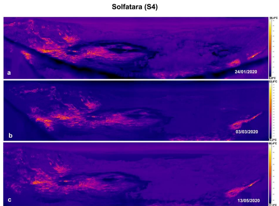
Figura 3.2.2 - Fotocomposizione di immagini termiche riprese dal punto stazione S2 di Figura 3.2.1d1, relative al 24/01/2020, 03/02/2020 e 13/05/2020.
