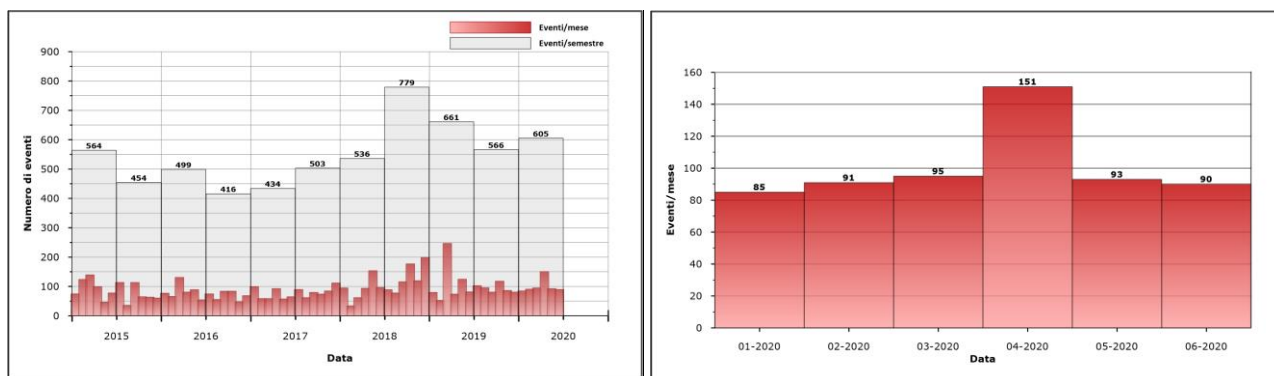
Figura 1.1.3 – Frequenza di accadimento dei terremoti vesuviani nel corso degli ultimi 5 anni (a sinistra) e del primo semestre 2020 (a destra).
