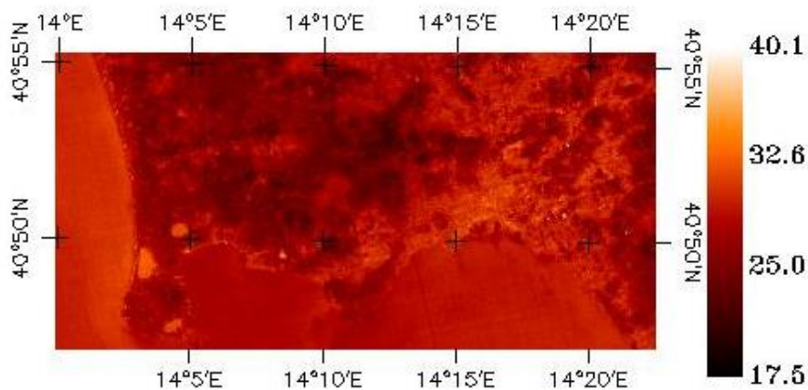
Figura 3.3.5 - Mappa di temperatura superficiale relativa al dato LANDSAT8 acquisito alle 20.46 UTC del 30 giugno 2020.
