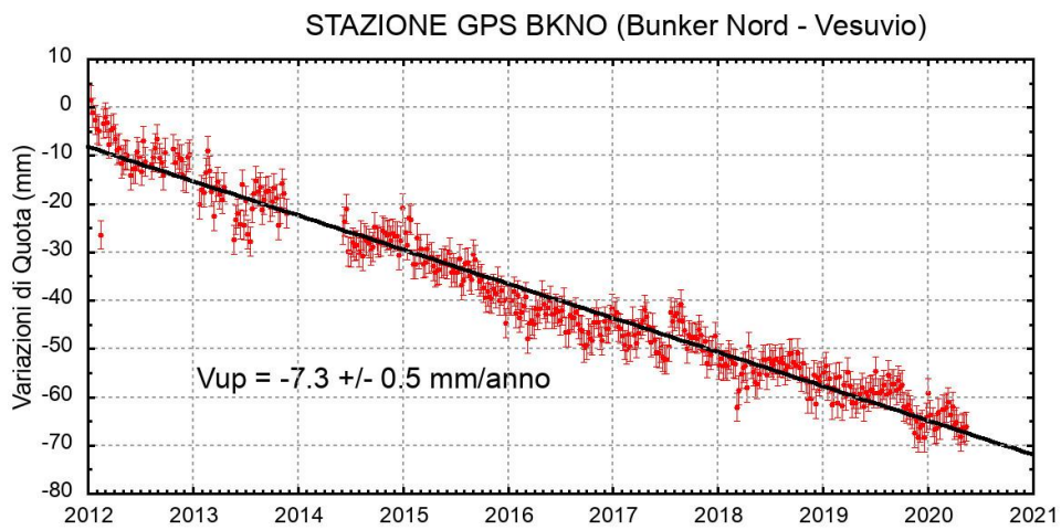
Figura 2.1.3 - Serie temporale delle variazioni settimanali in quota della stazione di BKNO (Vesuvio) da gennaio 2012 a giugno 2020.
