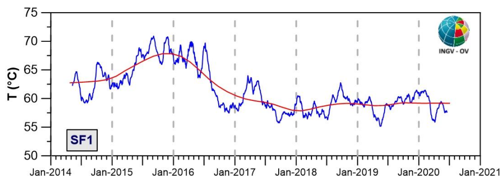
Figura 3.1.4 - Stazione Solfatara (SF1). Serie temporale delle medie mensili dei valori di temperatura massima rilevati nell'immagine IR destagionalizzata mediante applicazione dell'algoritmo STL.
