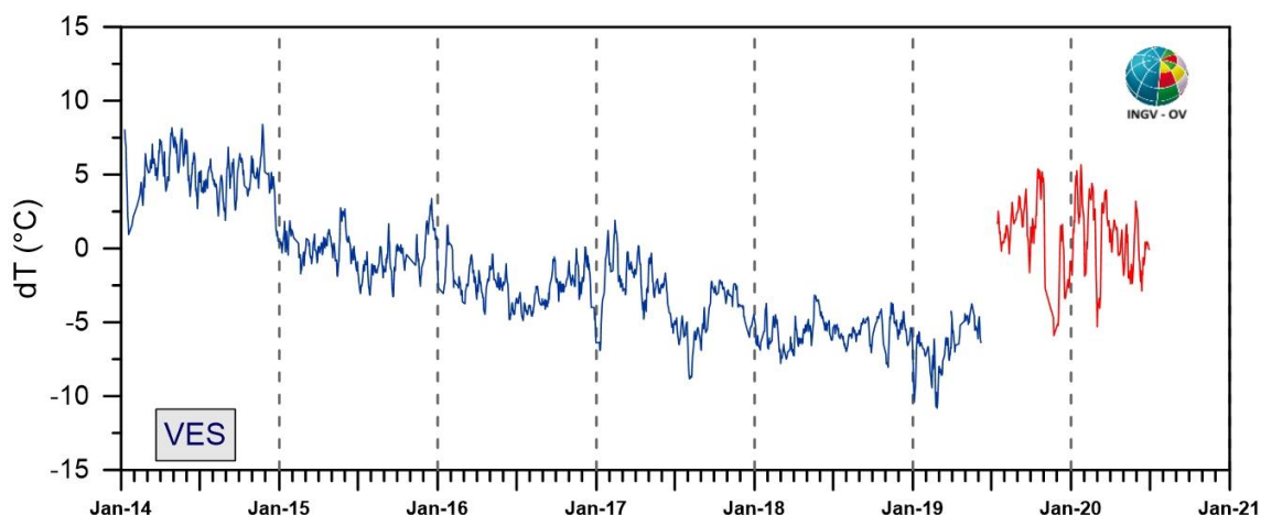
Figura 3.1.3 - Stazione Vesuvio: Serie temporali dei valori di temperatura massima giornaliera rilevata nelle immagini IR destagionalizzate mediante applicazione dell'algorithmo BR [medie settimanali termocamera 320x240 (blu); medie settimanali termocamera 640x480 (rosso)].
