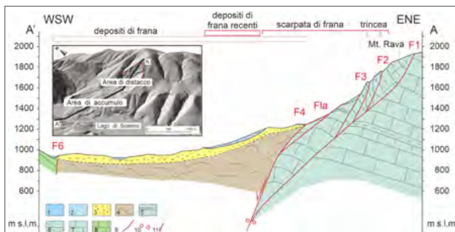
Figura 3. Sezione geologico-geomorfologica della frana di Scanno che mostra la connessione della scarpata di frana con la zona di faglia (Difesa-Monte Genzana), caratterizzata dall'intersezione di piani di faglia ad alto angolo (F1, F4) e piani di faglia a basso angolo (Fla). Nel riquadro è riportata la traccia della sezione. Legenda: 1) Depositi fluviali e di versante; 2) Depositi di frana recenti; 3) Depositi della frana di Scanno; 4) Rocce pelitico-arenacee; 5) Rocce argilloso-marnose; 6) Calcari marnosi; 7) Calcari e calcari marnosi; 8) Calcari; 9) Faglia; 10) Cinematica trascorrente; 11) Cinematica diretta
