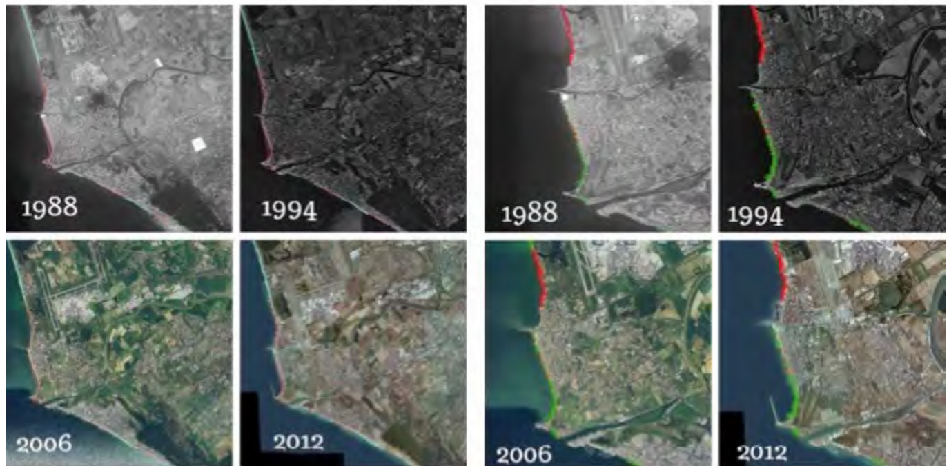
Figura 2a. Il delta del Tevere - Variazione linea di riva (fotoaeree 1988, 1994, 2006 e 2012)
