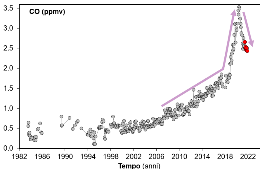
Figura 4.9 - Variazioni della concentrazione di monossido di carbonio (CO) misurato alla fumarola BG a partire dal 1983. In rosso sono evidenziati i campioni relativi al secondo semestre 2021. In generale alti contenuti di CO caratterizzano sistemi vulcanici ad elevata temperatura mentre fumarole alimentate da sistemi idrotermali mostrano concentrazioni più basse, in tali sistemi un aumento delle concentrazioni di CO può riflettere un incremento delle condizioni di temperatura e pressione.
