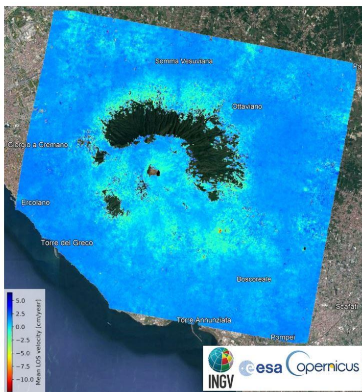
Figura 2.3.1 - Mappa della velocità media di deformazione nella linea di vista del sensore (Sentinel-1A/B) (03.01.2021-29.12.2021) per l'area Vesuviana. Dati IWS - TOPS mode, orbite discendenti (22), swath 1.
